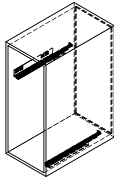
2. Расположение направляющих
